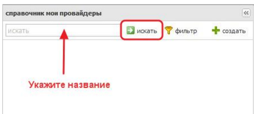
Рис. 6. Поиск провайдера
